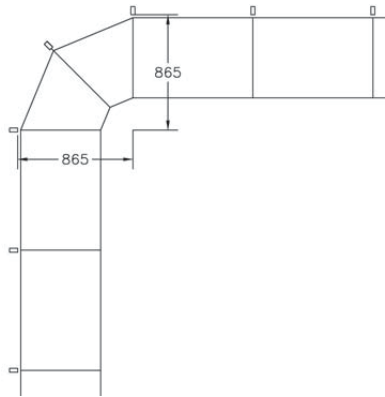
2x45 asteen kulman mitoitus pohjakuvassa
