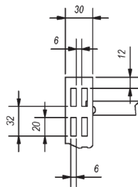
Säätöputkien reijityksen mitoitus
