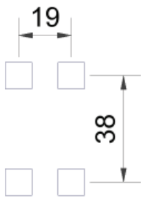
Reikätaustan reijityksen mitoitus Reijän koko 9,5x9,5mm
