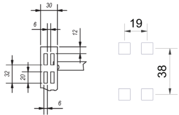
Säätöputken reikien mitoitus Reikätaustan mitoitus Reiän koko 9,5 x 9,5 mm
