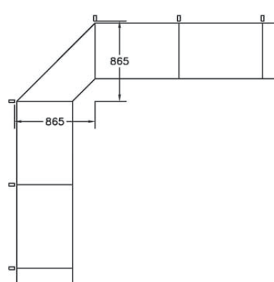
90 asteen kulman mitoitus pohjakuvassa
